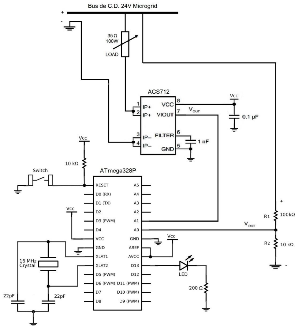
Figura 4.19. Diagrama de conexión entre MCU y sensores.
