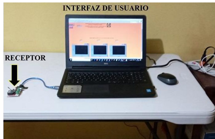
Figura 5.26. Receptor implementado.
